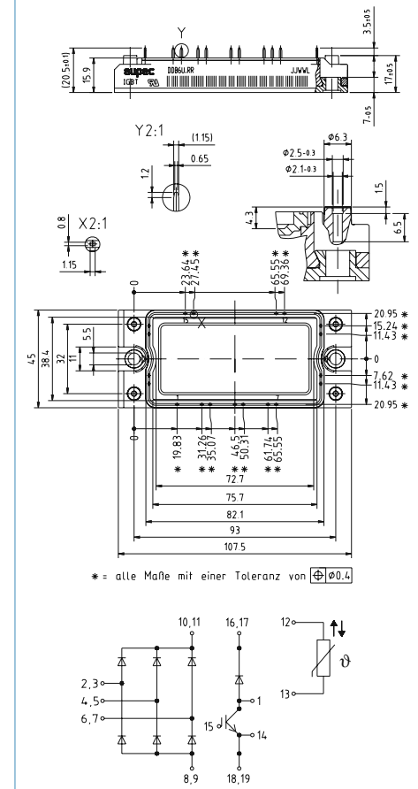
EconoBRIDGE™ Rectifier 2
