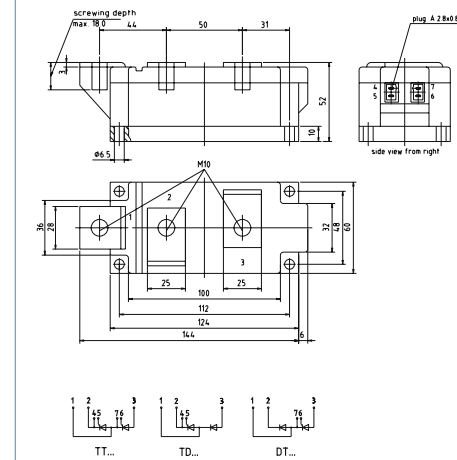
60 mm TP60
