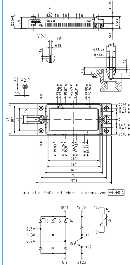
EconoBRIDGE™ Rectifier 2
