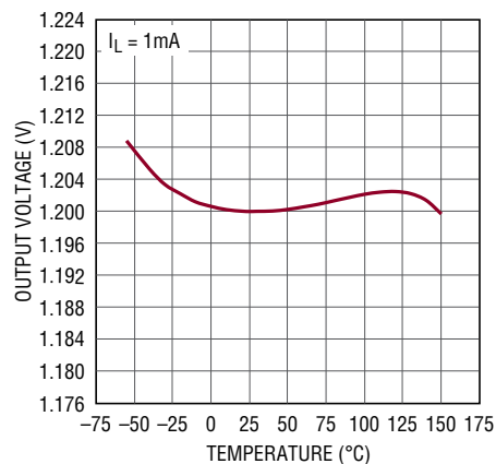
LT3065-1.2 Output Voltage
