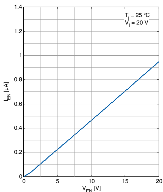
EN Pin Input Current versus EN Pin Voltage V_{\text{EN}}
