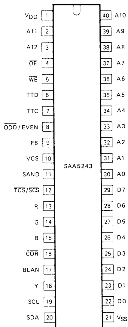
Fig.2 Pinning diagram.
